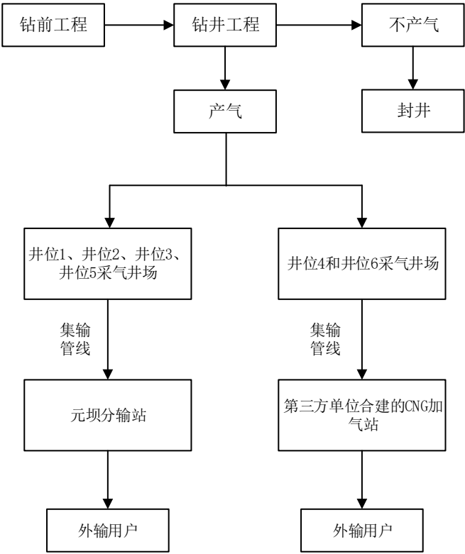
图 3.5-1 本项目天然气开采总体工艺流程
