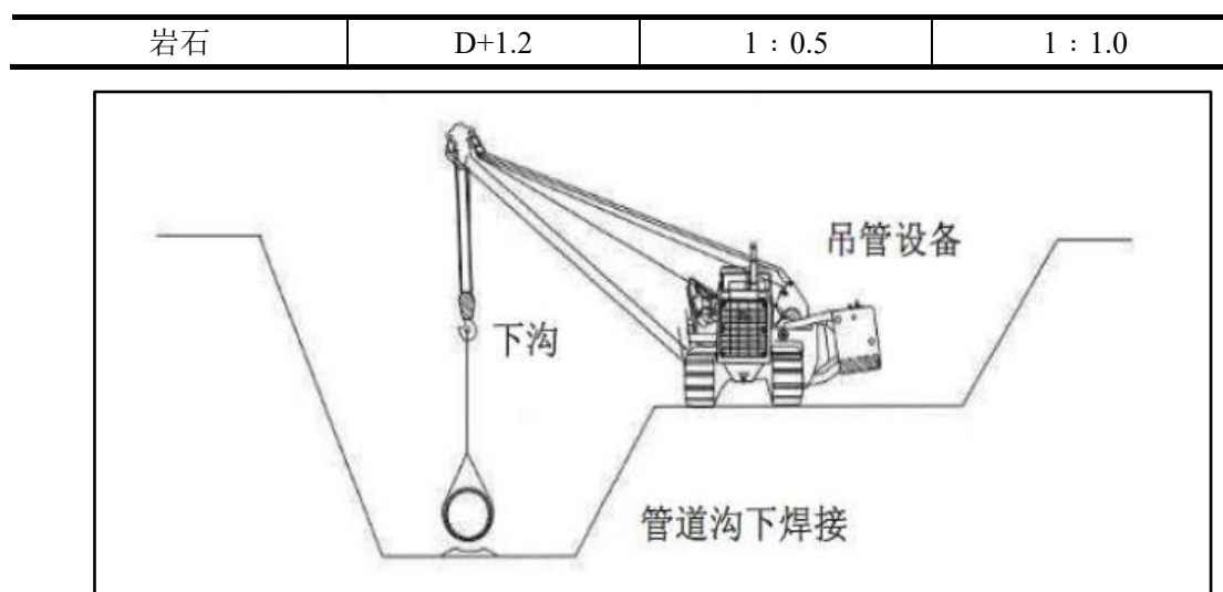
图 4.1-16 管道下沟施工示意图
