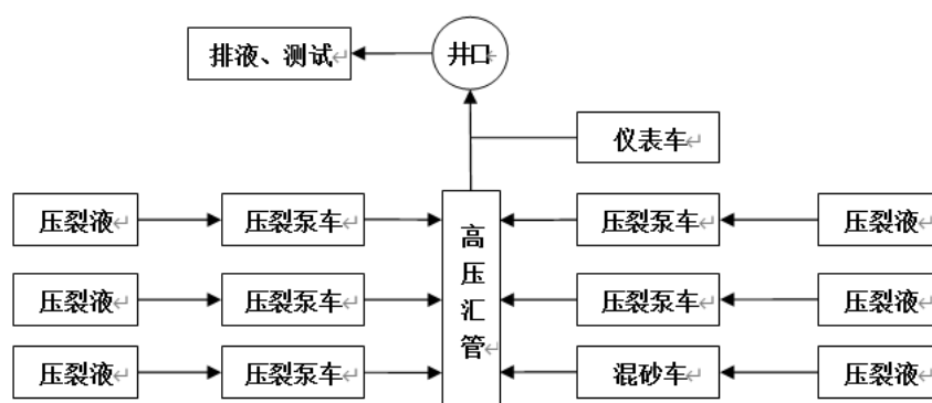
图 3.5-8 加砂压裂作业示意图
