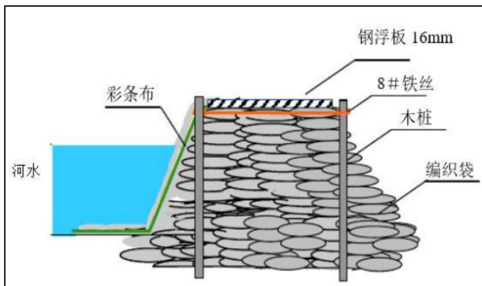
图 4.1-13 围堰施工工艺示意图
