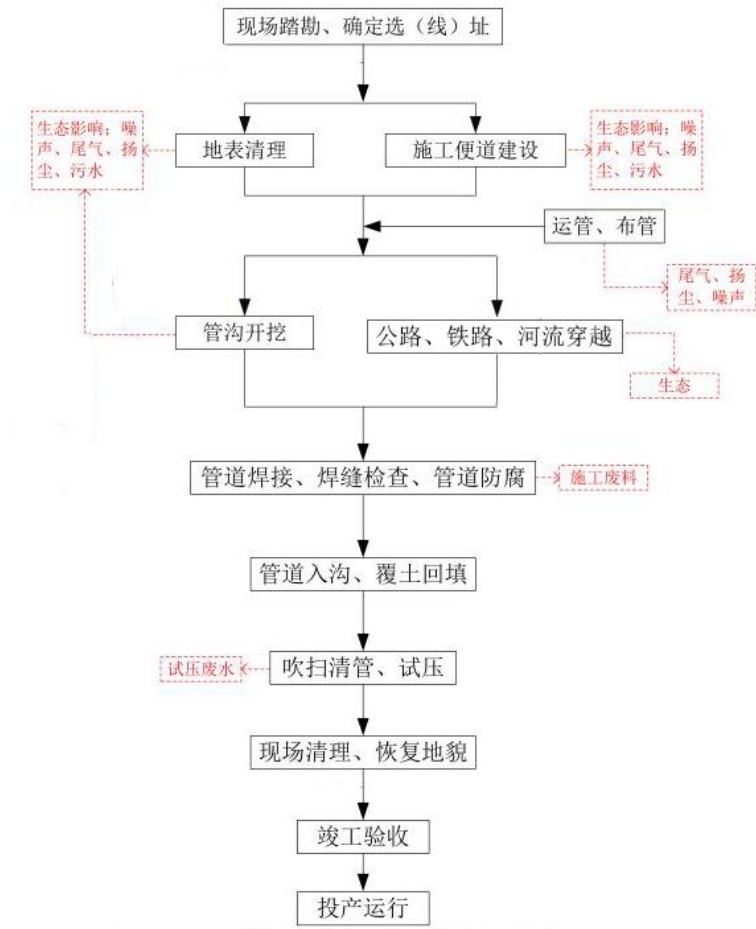
图 4.1-10 管线施工作业流程及产污节点图
