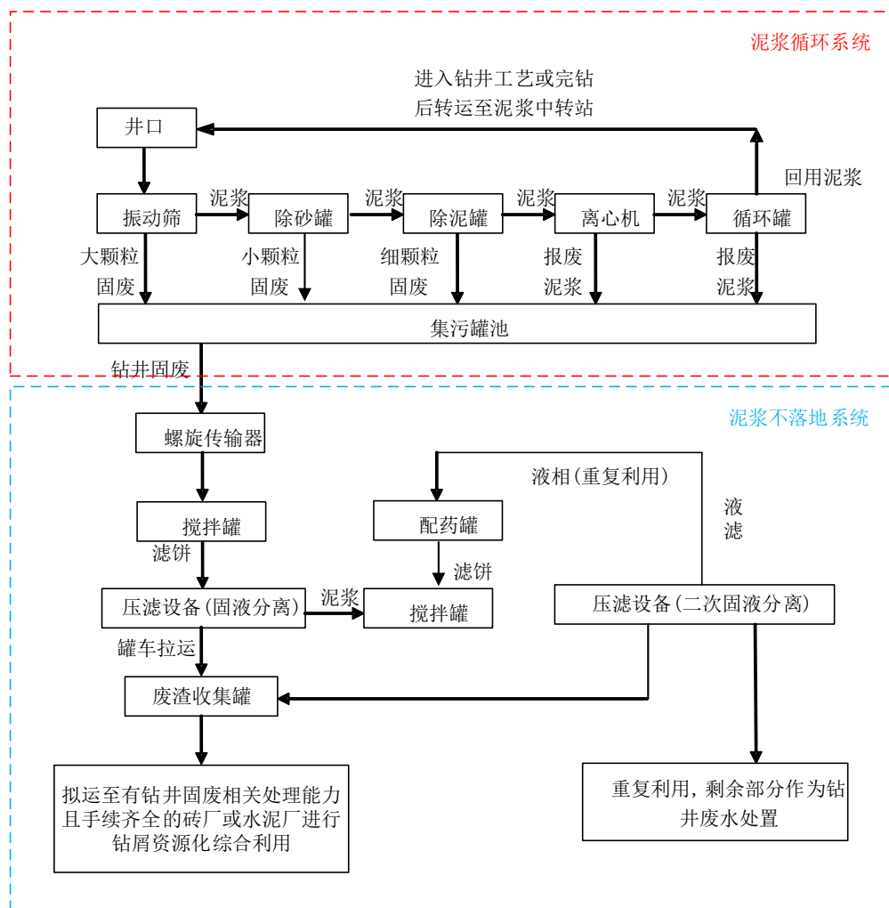
图 12.1-1 工艺联动运行示意图
