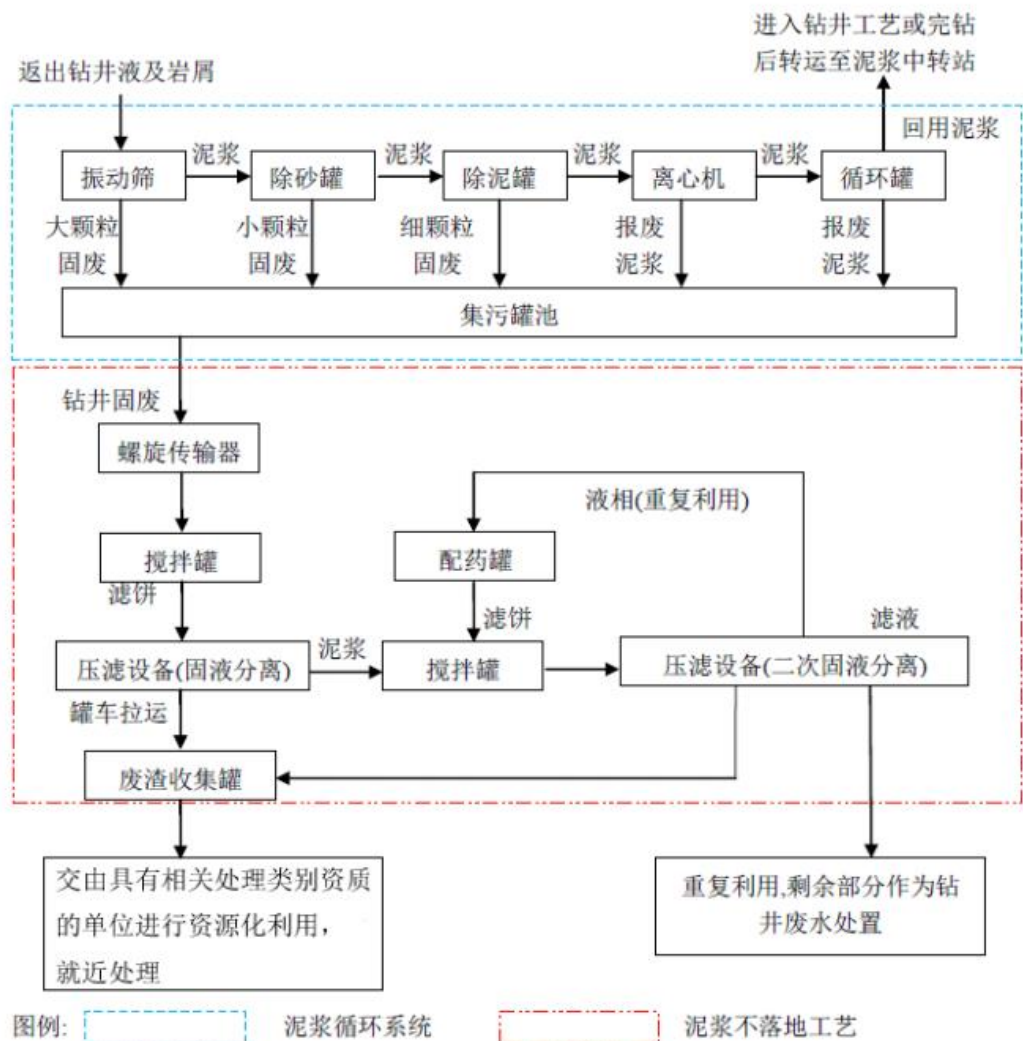
图 4.4-1 泥浆不落地工艺流程图
