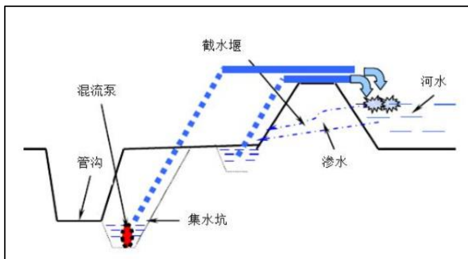
图 4.1-14 排水施工工艺示意图
