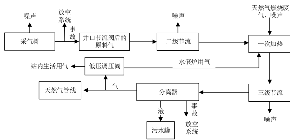
图 4.2-1 采气井场工艺流程图
