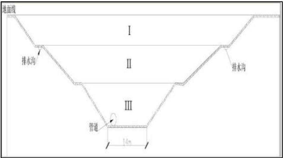
图 4.1-15 挖沟施工工艺示意图
