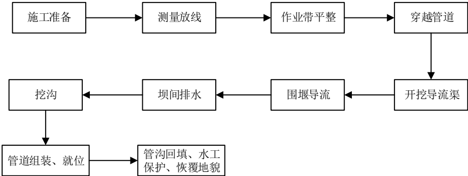
图 4.1-11 穿越河流施工流程示意图
