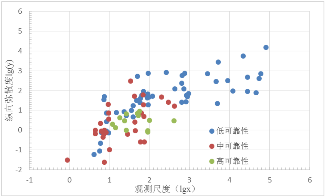
图 8.14-1 纵向弥散度对观测测度、数据根据可靠性分类：弥散系数=弥散度*渗流速度
