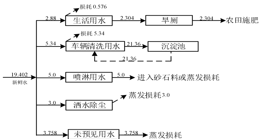
图 2-1 项目水平衡及废水处理图 ( \text{m}^3/\text{d} )
